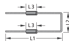
Typ/Type G/*GS
